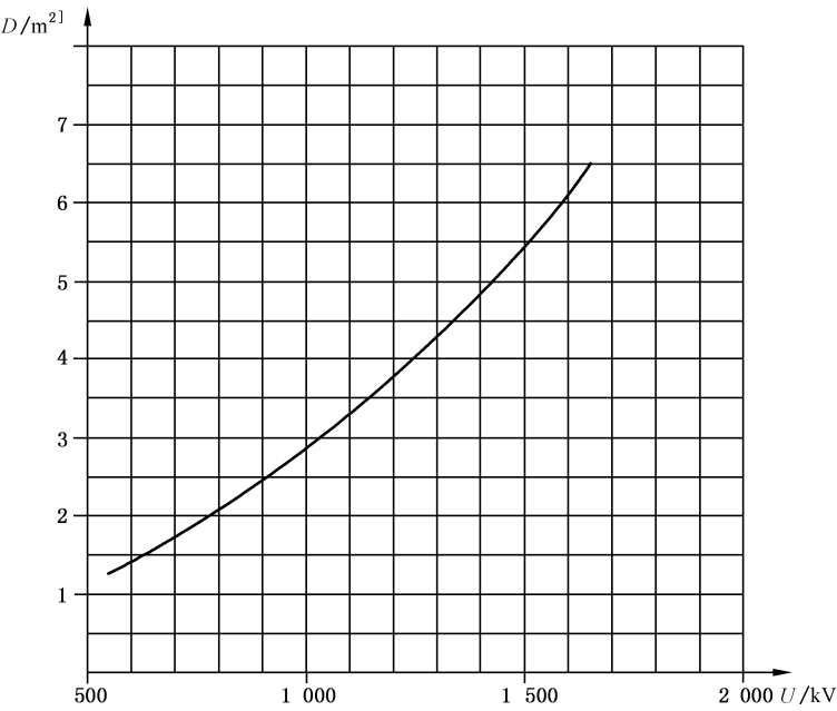
图 5 根据额定操作冲击耐受电压的相对地空气间隙
