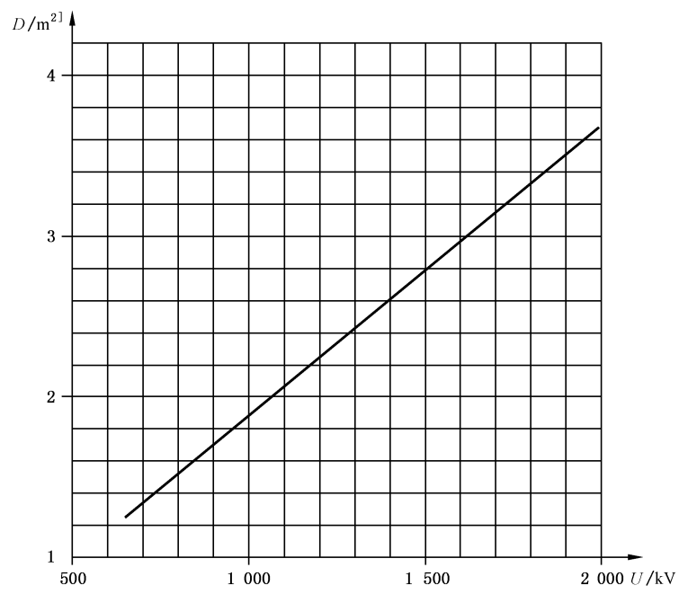
图 7 根据雷电冲击耐受电压的空气间隙
