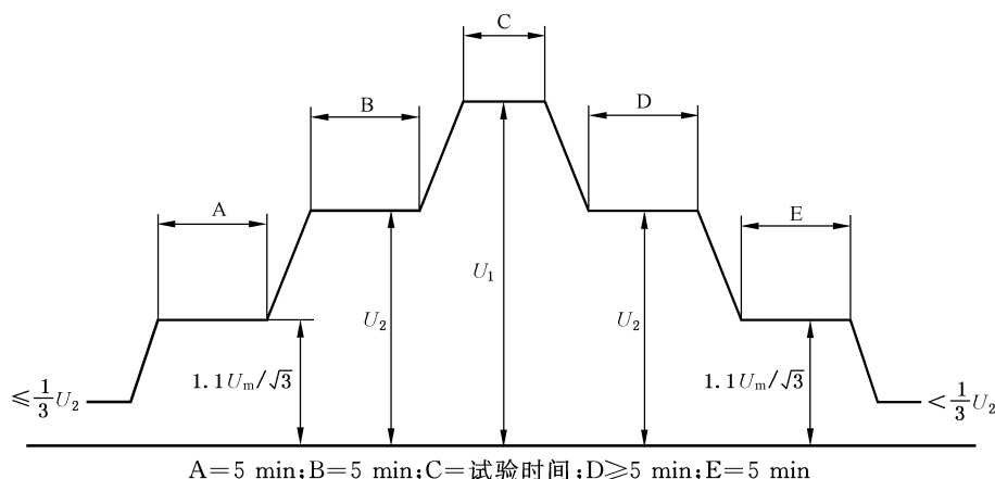
图 1 施加对地试验电压的时间顺序
