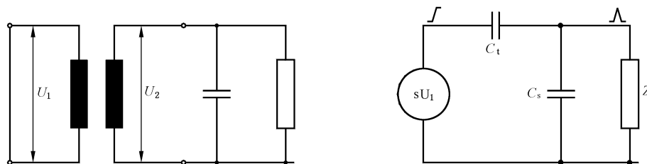
图 B1 过电压电容传递的等值电路
