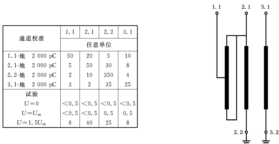
图 A3 用“多端子测量”和“读数分布对比图”的方法确定局部放电源的位置
